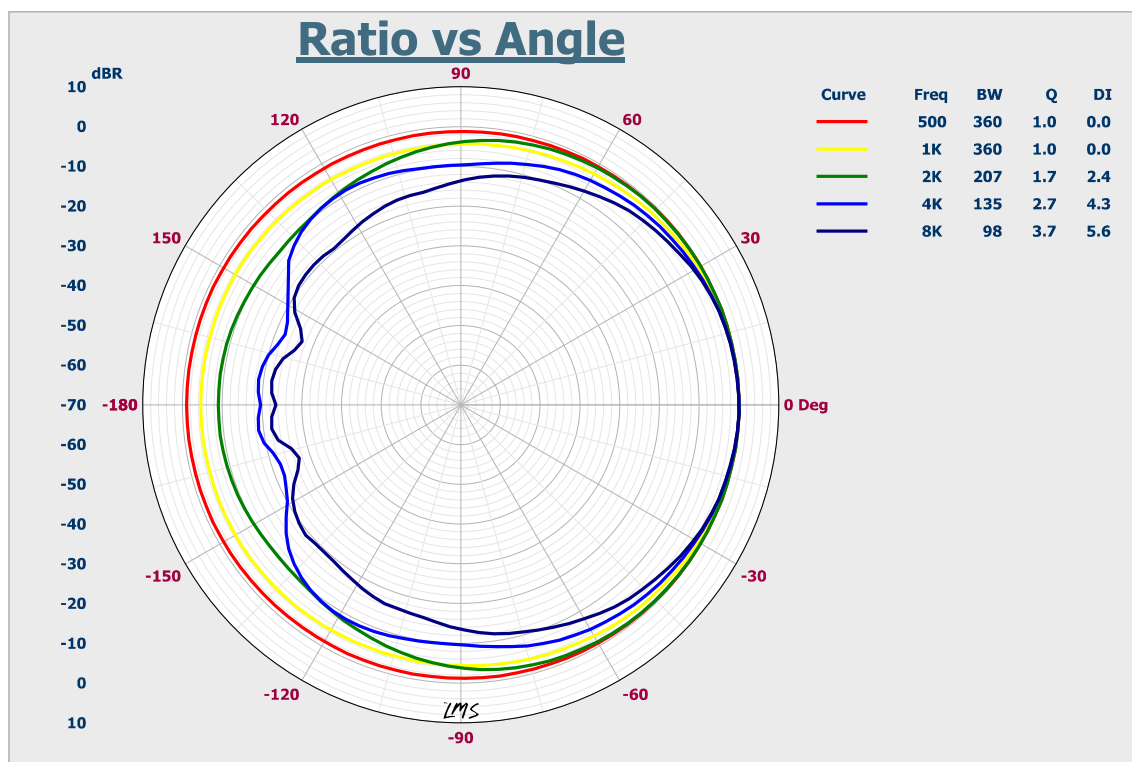
Круговая диграмма направленности громкоговорителя LPA-40CA (цвет черный)
